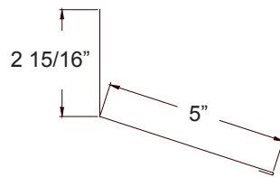
"Endwall Flashing"
