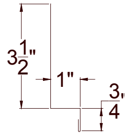
WSW4 Sidewall
