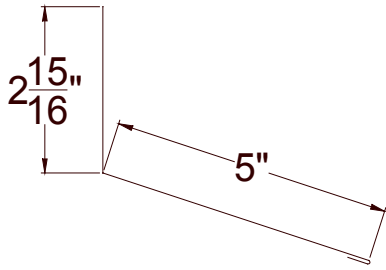
WEW2 Endwall
