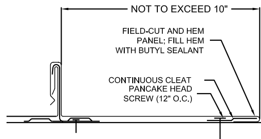
FASCIA EDGE
